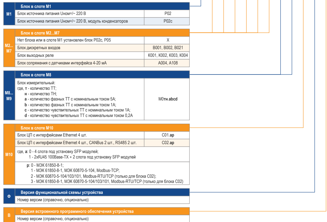
Рисунок А.1 – Код заказа устройства «ЮНИТ-М314-АРНТ» (Исполнение I)
